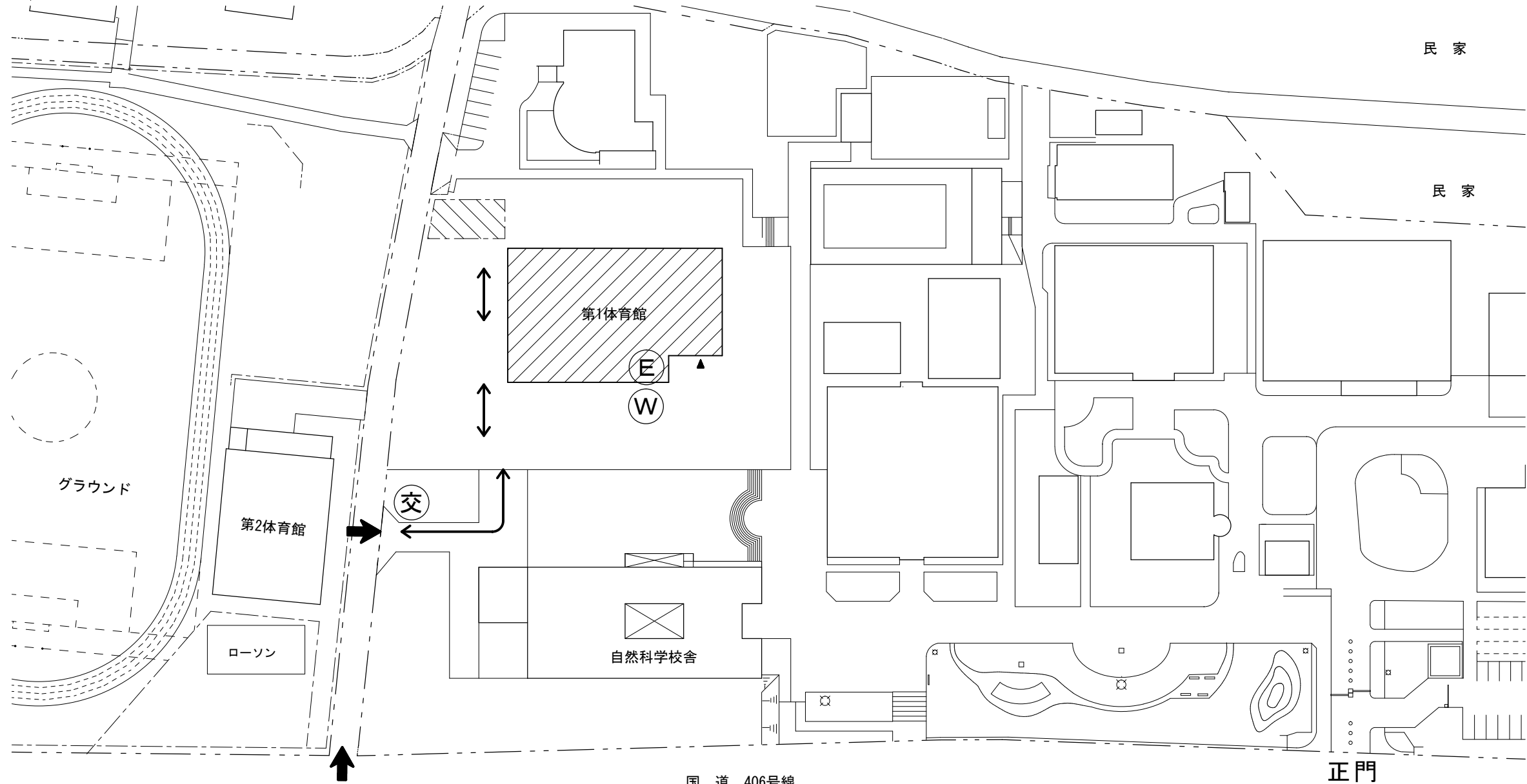
本工事建物周辺配置図 S=1/1000
